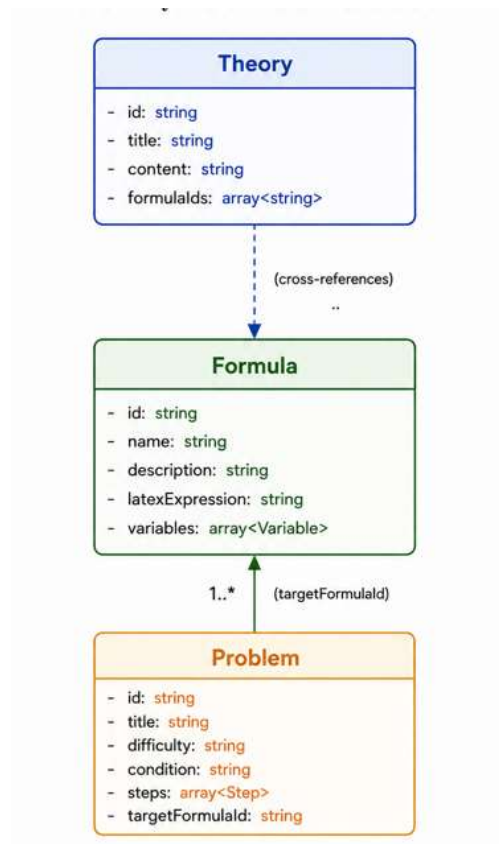
Рисунок 2.7 UML-діаграма класів для основних сутностей бази знань SciLearn
