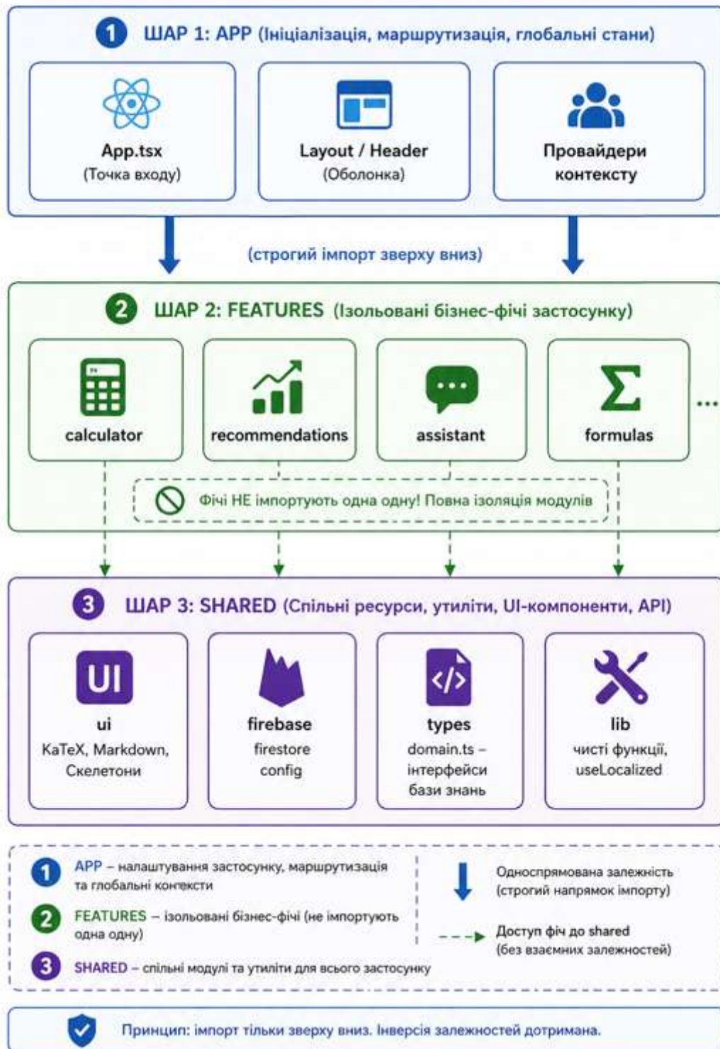
Рисунок 2.6 Загальна структурна схема архітектурних шарів та односпрямованих залежностей за методологією Feature-Sliced Design у системі SciLearn
