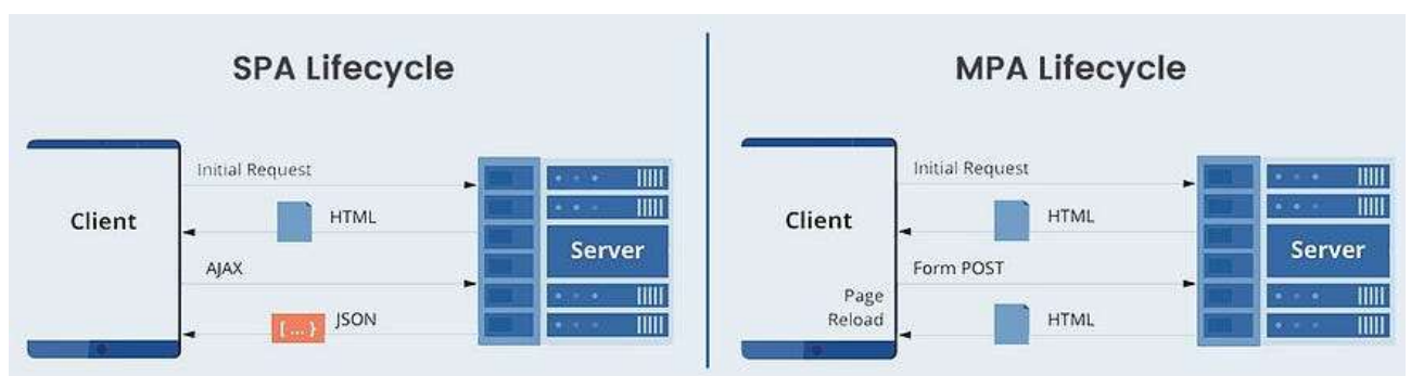
Рисунок 1.1.Схема взаємодії між клієнтом та сервером у архітектурних моделях МРА та SPA
