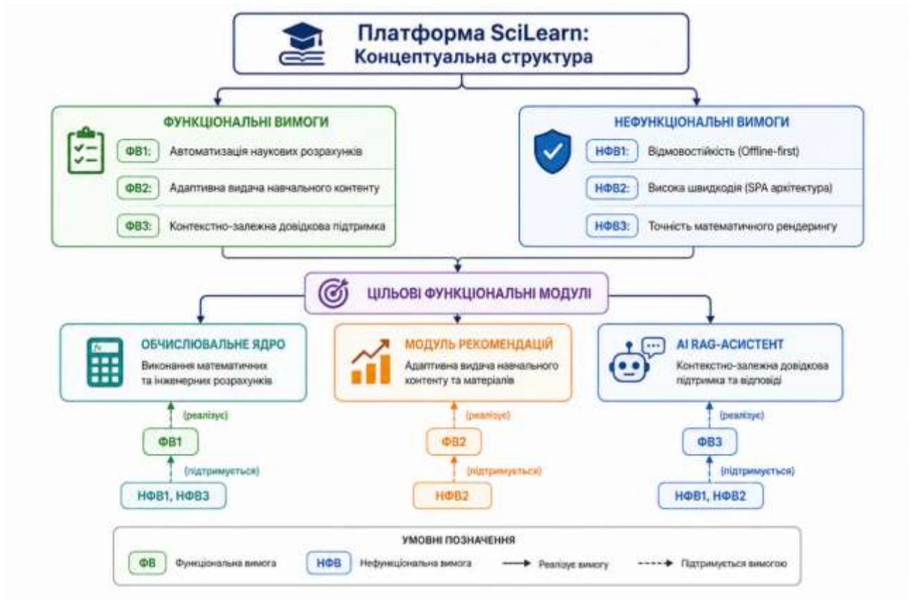
Рисунок 2.1 Схема концептуальної структури вимог та зв'язків між функціональними модулями платформи SciLearn
